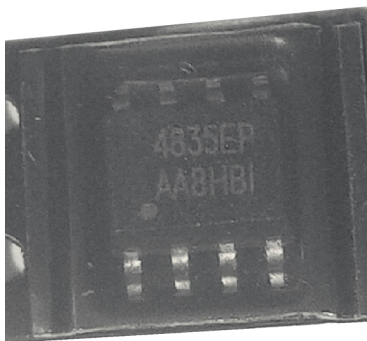
IC 4835EP
