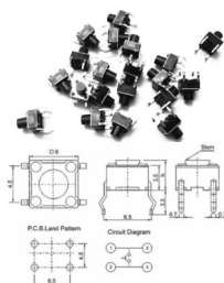
Pulsador 6 X 6 X 4.5mm Na Dip-4 Serie Tc-6615
