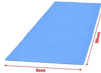
Thermal Pads 6.0w/m-k 10x3cm 1.5mm, Almohadilla Térmica De Silicona
