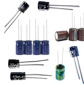
Condensador Electrolítico De Aluminio Dip 100uf 16v
