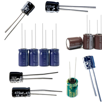
Condensador Electrolítico De Aluminio Dip 1000uf 10v
